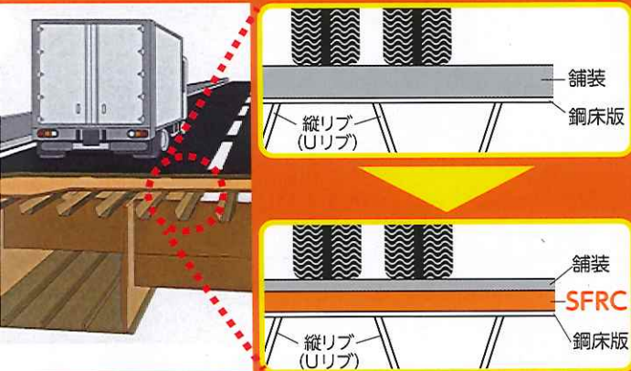
断面構成図
